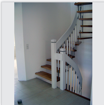
Alco, Schody bolcowo-dystansowe ½ zabiegu. Materiał: stopnie wykonane z drewna jesionowego, kolor naturalny; pozostałe elementy wykonane z drewna bukowego w kolorze RAL 9003. Wypełnienie balustrady: tralka pionowa – połączenie stali nierdzewnej z drewnem.
