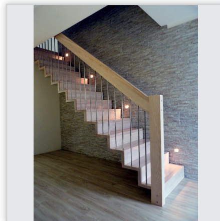
Alco, Schody dywanowe proste. Materiał: schody wykonane z drewna jesionowego zabielenego. Wypełnienie balustrady: tralka pionowa ze stali nierdzewnej.
